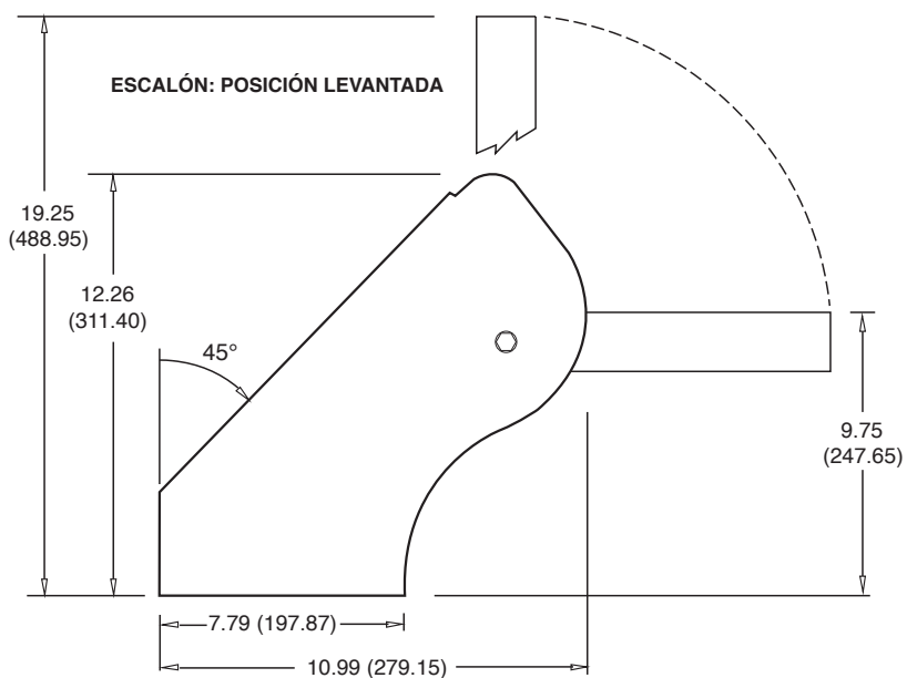
Vista lateral
